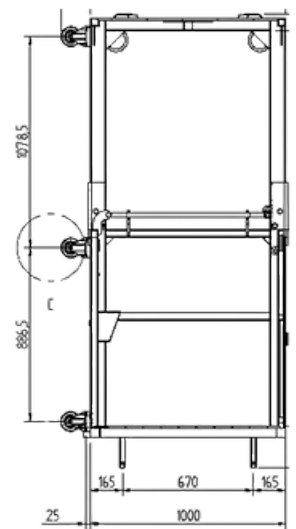
SEZIONE A-A
